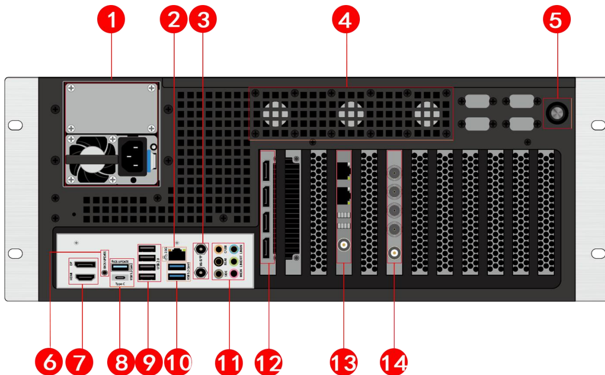
后面板
